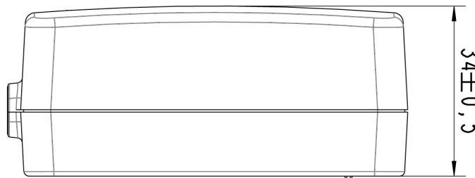
Primärstecker auswechselbar AC - plug exchangeable
